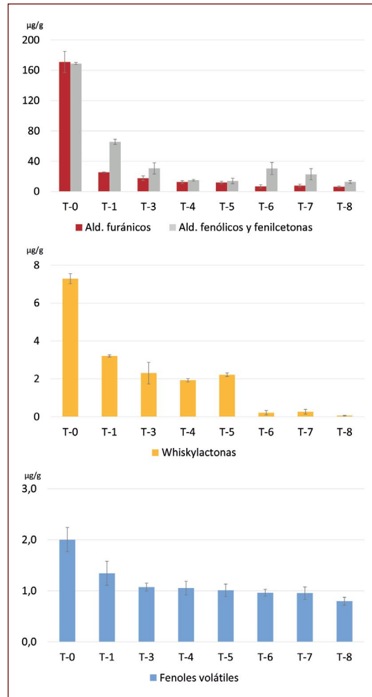
Figura 3. Compuestos volátiles ( \mu g/g) agrupados por familias procedentes de la madera de tinas de roble a lo largo de ocho años. Valores promedio y desviación estándar de las cuatro tinas.
